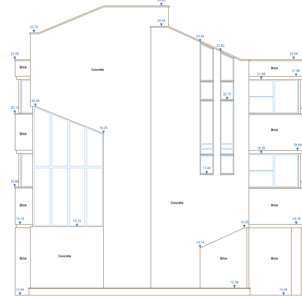
Elevation 4 Datum 11.00m
